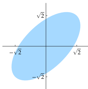
\mathbb{R}^2 中的椭球 E(2f_1, f_2) ，其中 f_1 = (\frac{1}{\sqrt{2}}, \frac{1}{\sqrt{2}}) ， f_2 = (-\frac{1}{\sqrt{2}}, \frac{1}{\sqrt{2}}) 。
