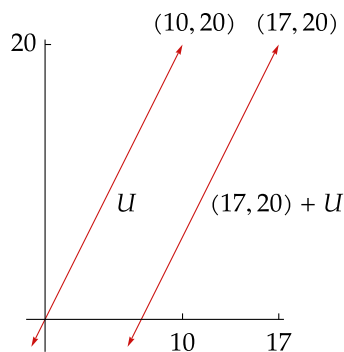
(17, 20) + U 平行于子空间 U .
